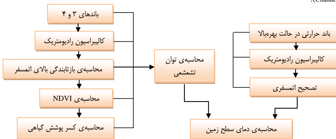
شکل (۲): نمودار گردش فرآیند دستیابی به دمای سطح زمین
